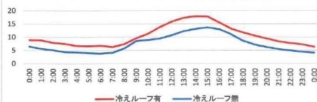
コンビニエンスストアの天井裏温度比較
